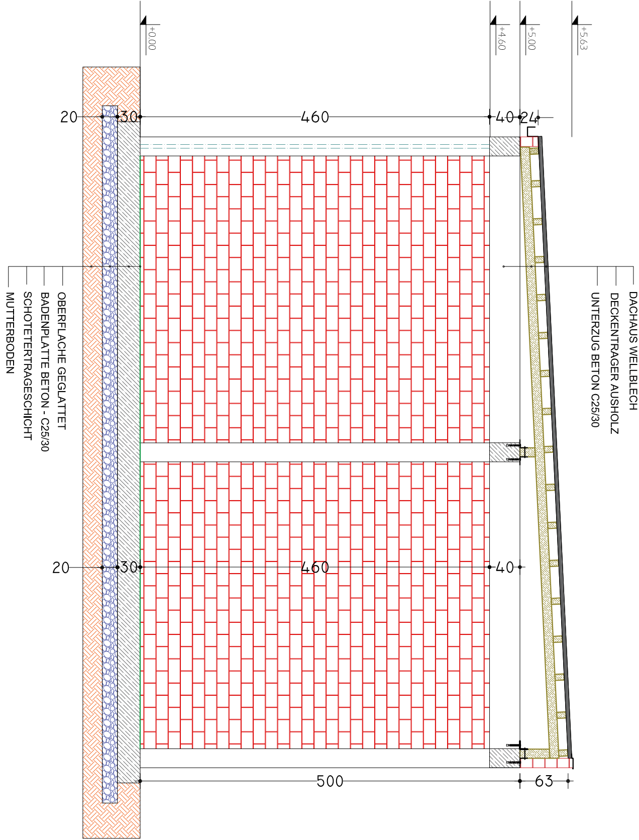
SCHNITT - "1-1"
