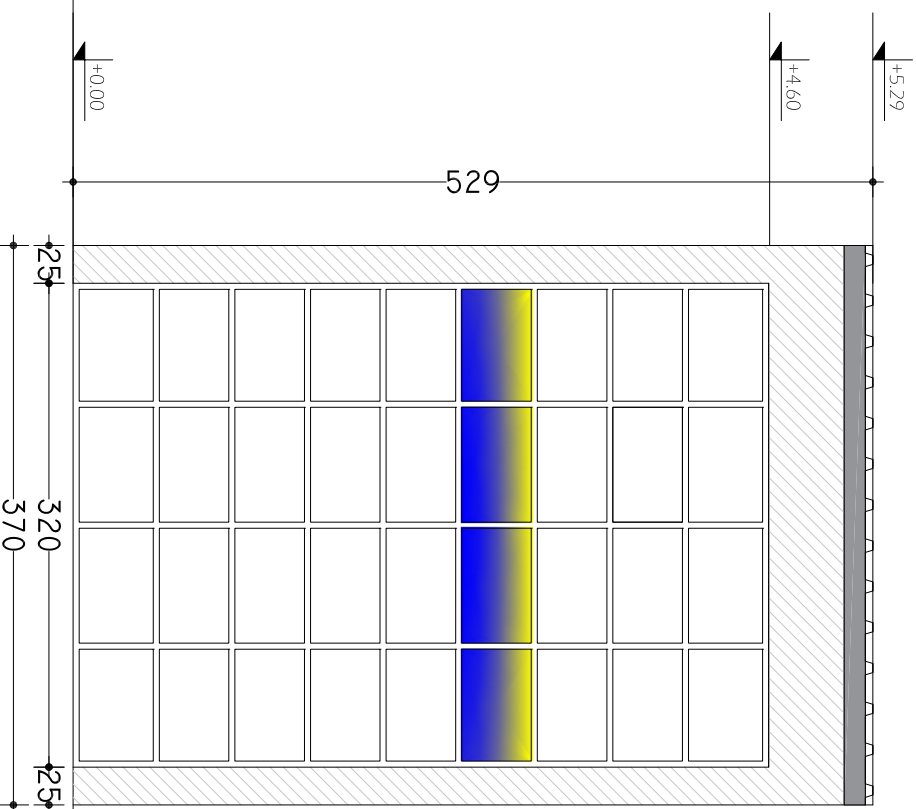
ANSICHT - 2
